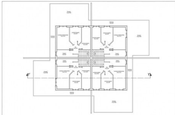
PLANIMETRIA PIANO PRIMO - SUPERFICI - Scala 1:100
