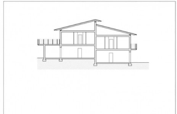
SEZIONE Y-Y - Scala 1:100
